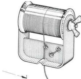
Figur 2. Vikleapparat
